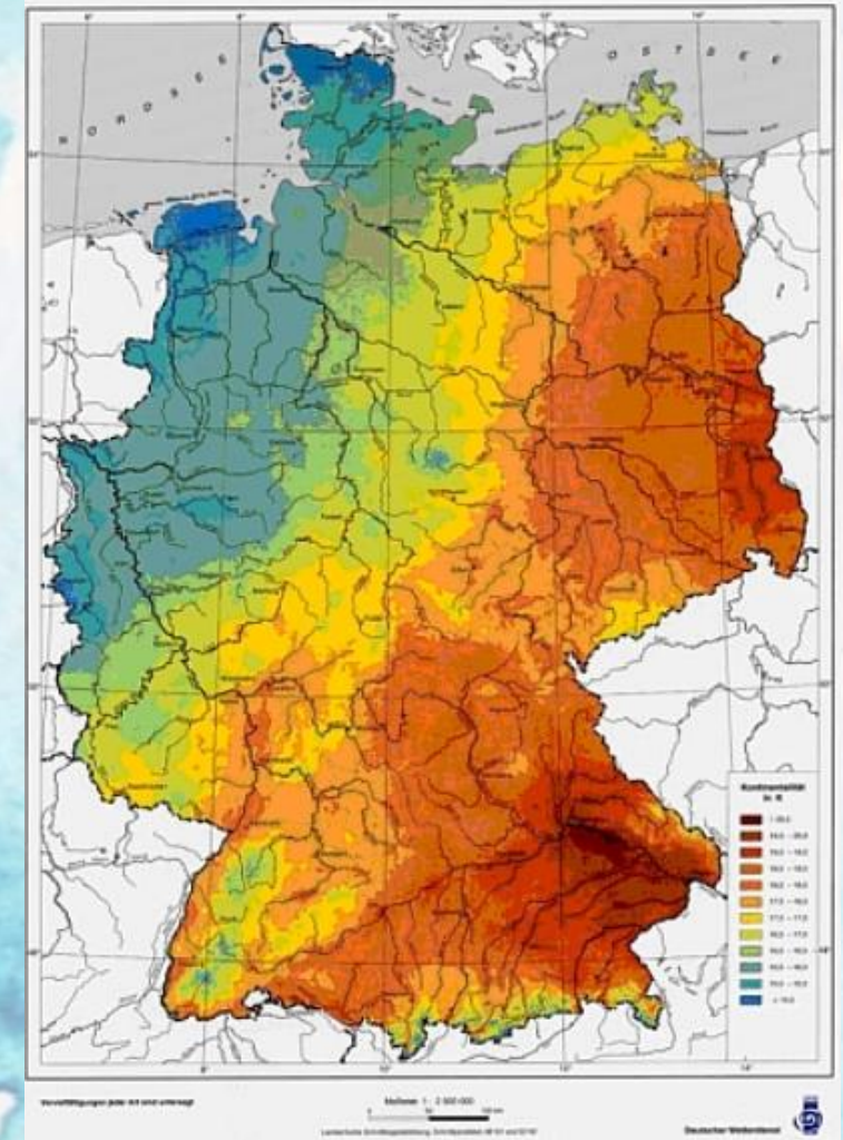
Klimaatlas: 1961-1990
